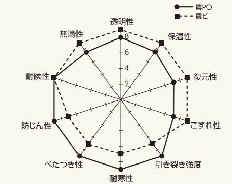
図2 農ビと農POの性能比較
