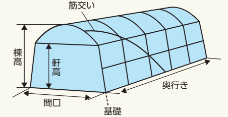
図1 ハウスの構造
